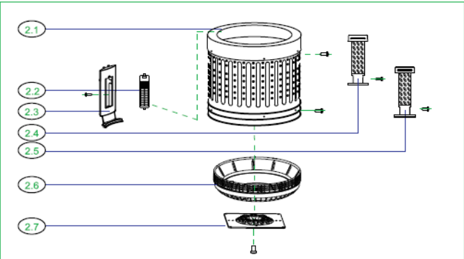
b: Spin Tub Subassembly
